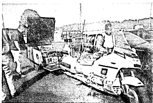
בתמונה מימין: אופנוע ההונדה לכל אורכו עם הציוד הנגרר. בתמונה משמאל: הנגרר ומערכת האנטנות.
